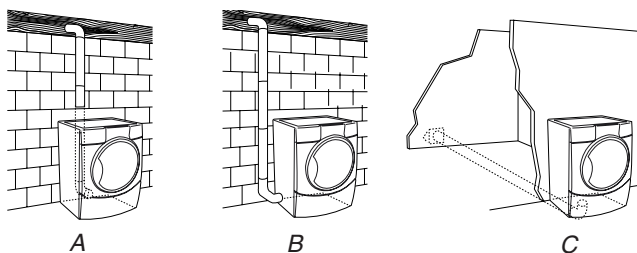
A. Instalación estándar con desviación de la ventilación en la parte posterior B. Instalación de ventilación lateral a la izquierda o a la derecha C. Instalación de ventilación inferior (no es apta para instalaciones de pedestal)
